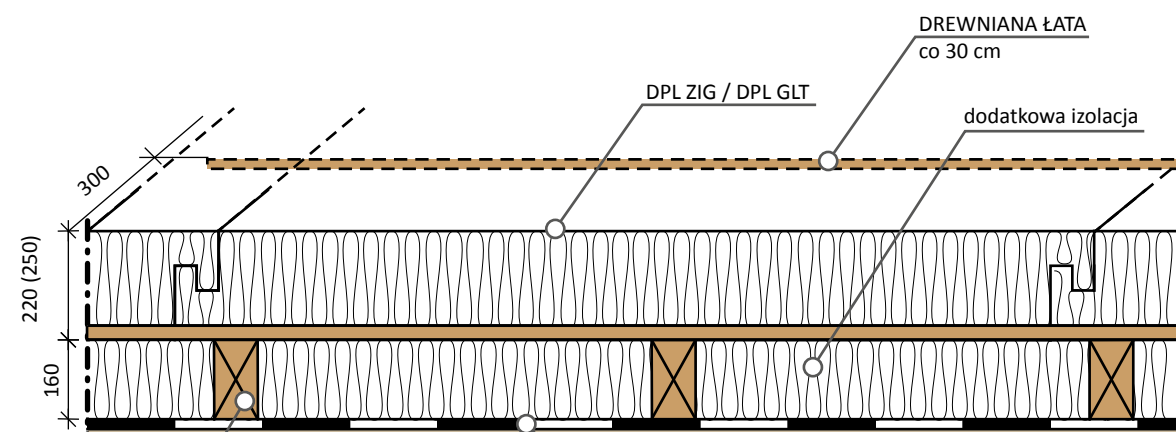
Rys. B Przekrój poziomy przez połac dachową z dodatkową izolacją międzykrokwową.
