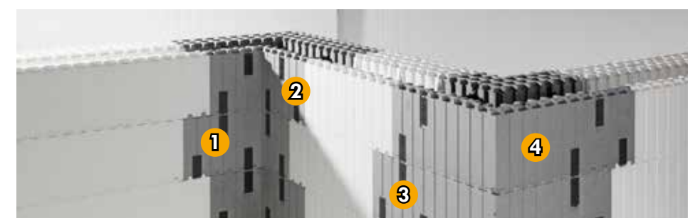
Schemat wykorzystania narożników, widok od wewnątrz budynku. Wykorzystane elementy: ① MCFU35 E90 LA, ② MCFU35 E90 RA, ③ MCFU35 E90 LI, ④ MCFU35 E90 RI.
