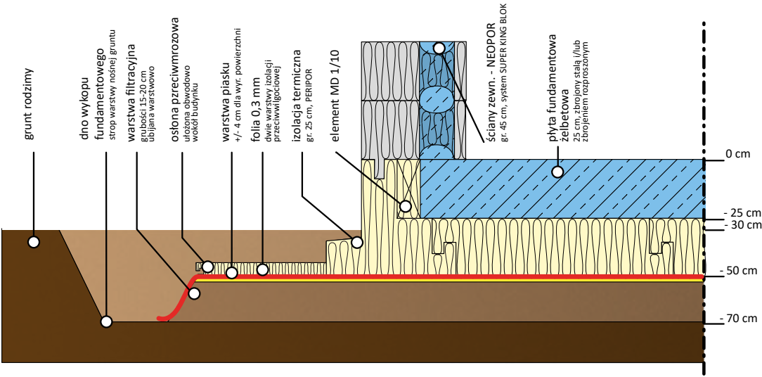
Rys. 1 Schemat wykonania fundamentu płytowego w wersji ze ścianami zewnętrznymi o szer. 45 cm (Super King Blok)
