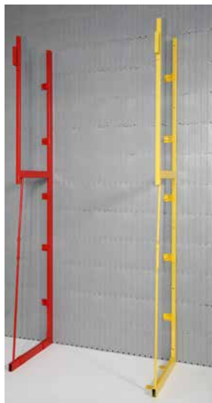
Stalowe podpory ułatwiają budowę ściany, kontrolę płaszczyzn z zachowaniem pionu. Podpory w kolorze czerwonym przystosowane są do montażu nadstawki o wys. 110 cm.
