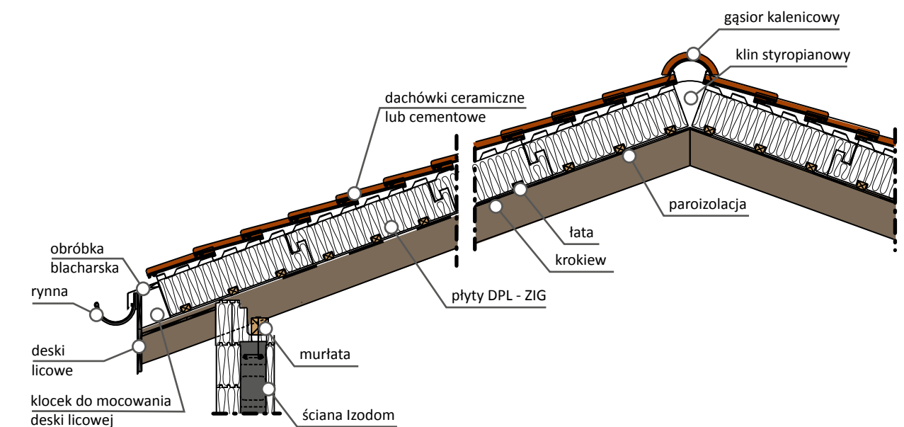
Rys. C Przekrój pionowy ilustrujący wariant pokrycia dachu dachówką - karpiówką.
