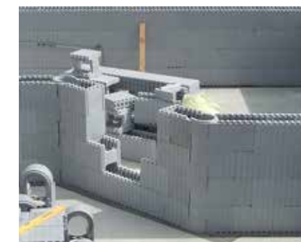
Uso de los componentes de bisagra para formar equinas con cualquier ángulo.
