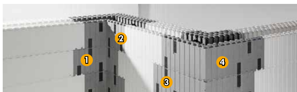
Esquema del uso de las esquinas, vista desde el interior de un edificio. Componentes usados: ① MCFU35 E90 LA, ② MCFU35 E90 RA, ③ MCFU35 E90 LI, ④ MCFU35 E90 RI.
